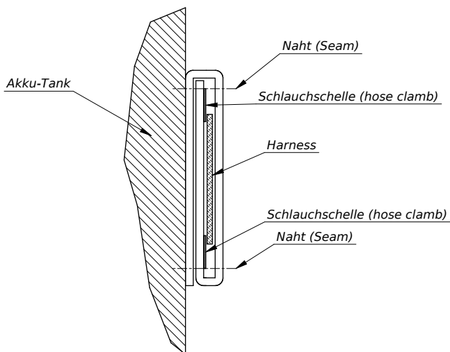
Figure 3.1: Gurtschlaufe
